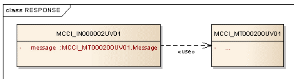
Figura 2 – Componenti della struttura MCCI_IN000002UV01.
